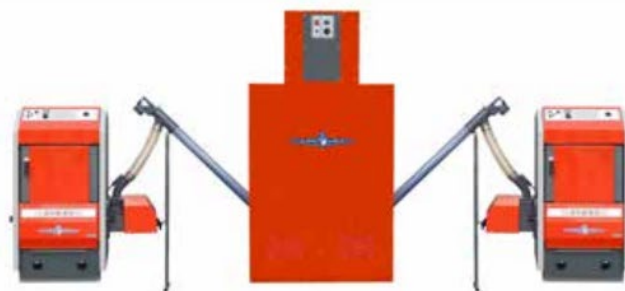
inštalácia APS 500 pre dva kotly
