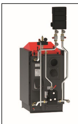
DC 32S + ATMOS F2 LADDOMAT
